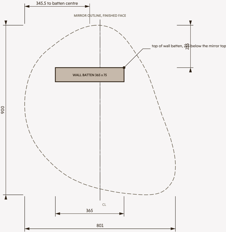
WALL SETOUT
